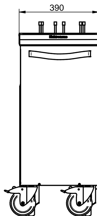
Ritning visar ETD 240-20 EC
