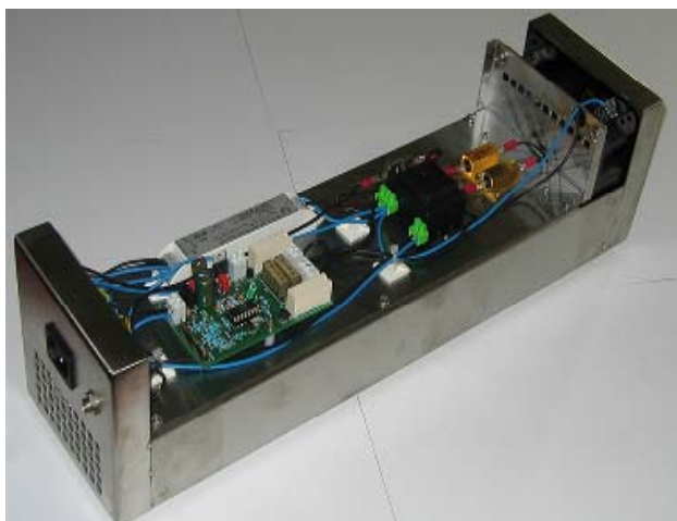
Luftrenaren med höljet avlägsnat
